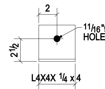
2 - ANGLES - a1395 (GR.-A36)
