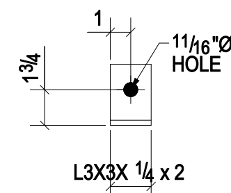
4 - ANGLES - a1475 (GR.-A36)
