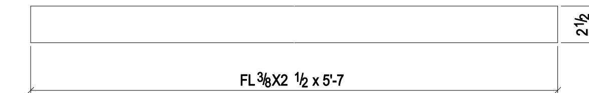
ONE - PLATE - p2086 (GR.-A36)
