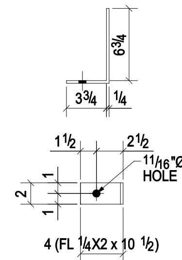
4 - BENT PLATES - p1542 (GR.-A36)
