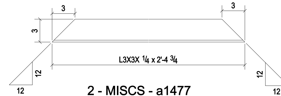
2 - MISCS - a1477 (GR.-A36)
