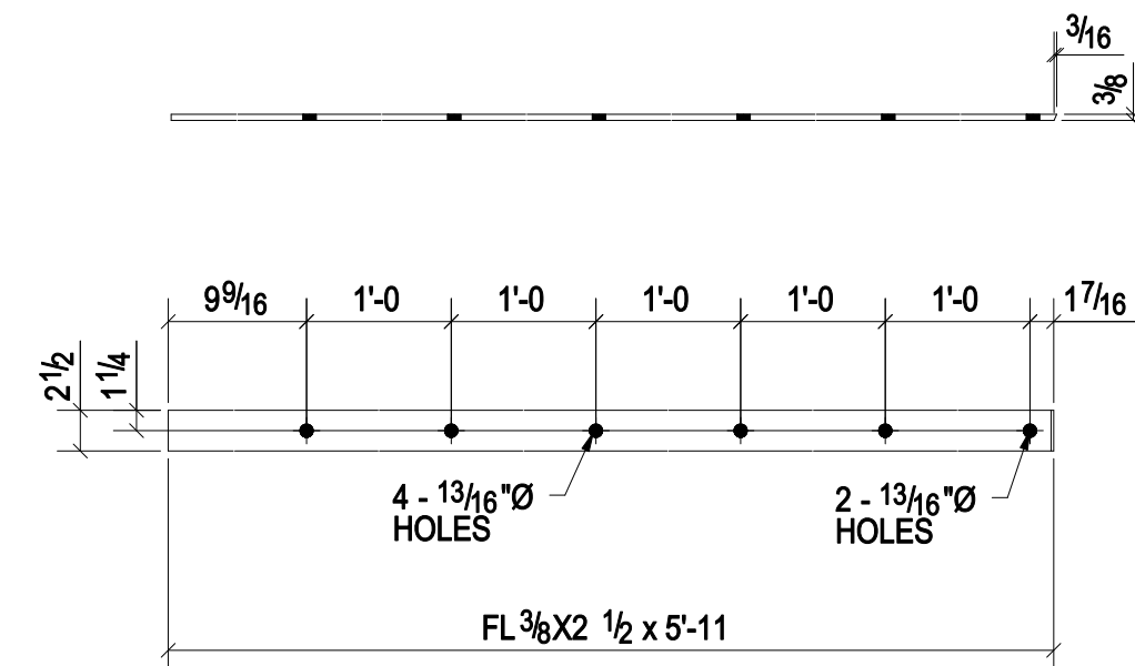
ONE - LADDER - p2458 (GR.-A36)
