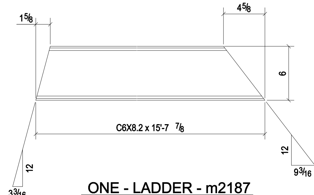
ONE - LADDER - m2187 (GR.-A36)
